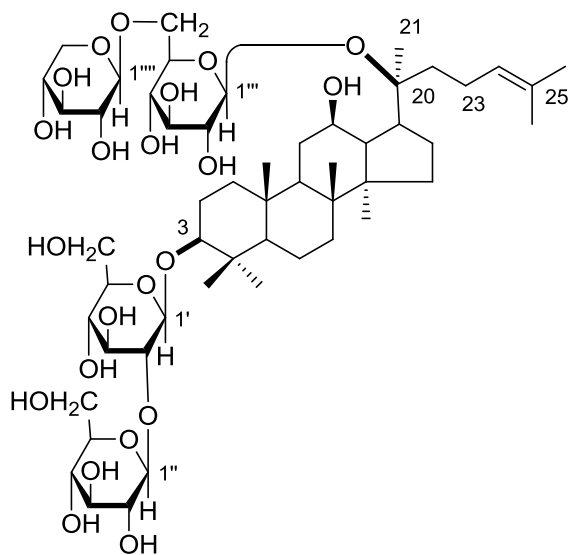
人参皂苷Rb 3
