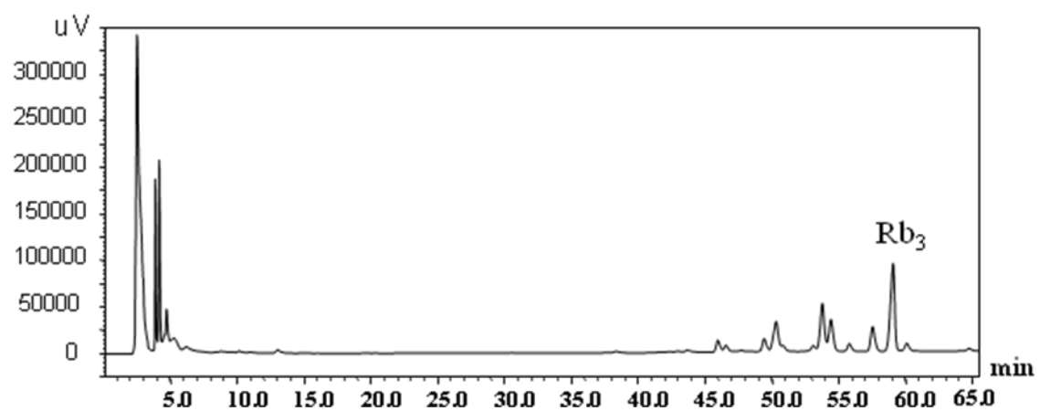
图A.3 三七花样品液相图
